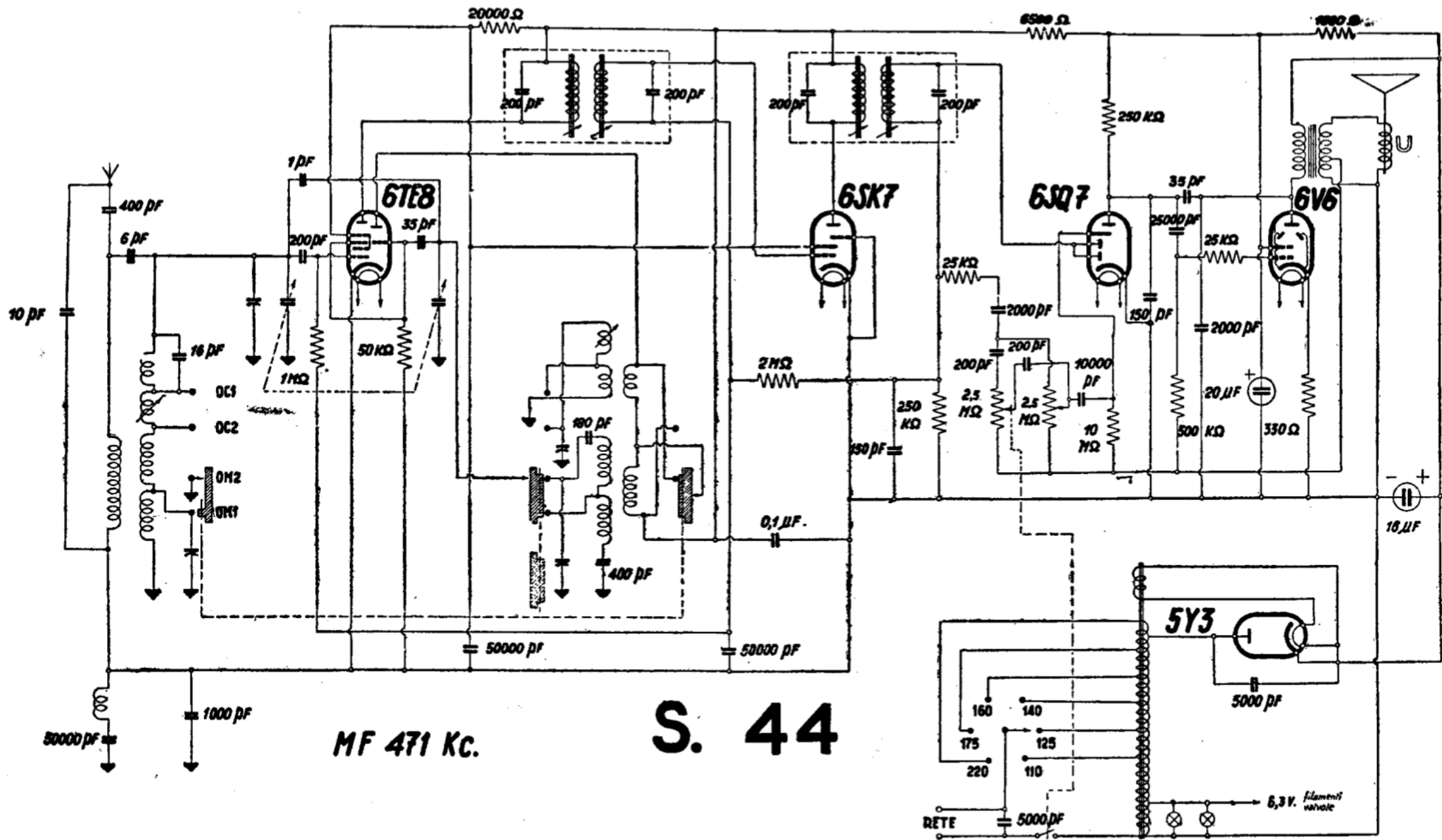
MAGNADYNE RADIO - Modd. S44, S106 e S441 - Lo schema è del mod. S44 - I modd. S106 e S441 hanno in più la presa fono ed il relativo commutatore. I modd. S105, S107 e S109 hanno in più anche l'occhio magico.
